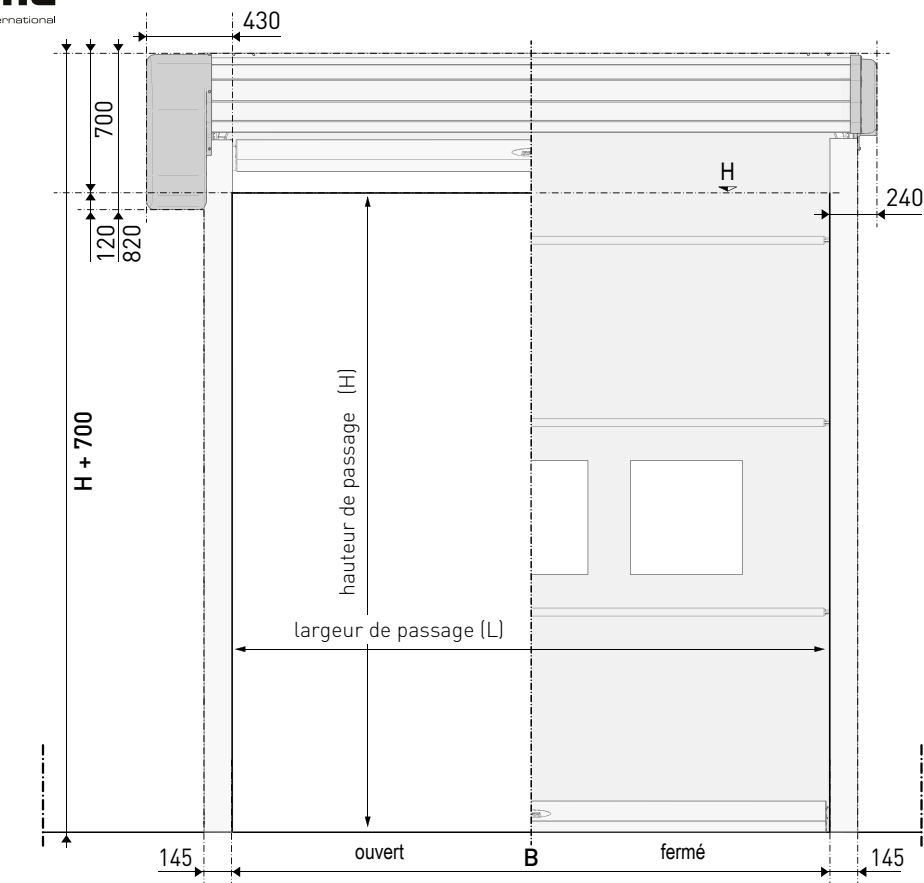
[ Côté entraînement ]
