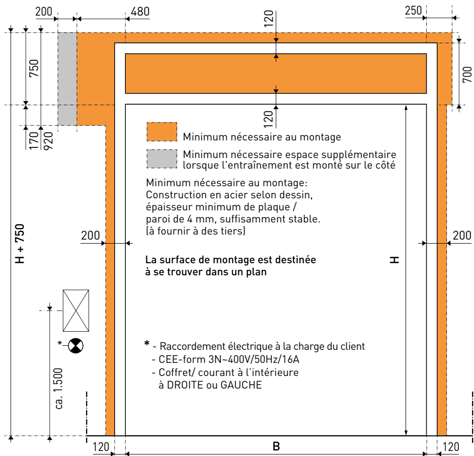
[ Côté entraînement ]
