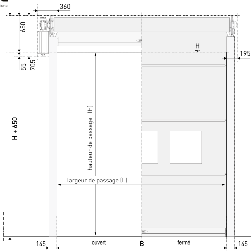
[ Côté entraînement ]
