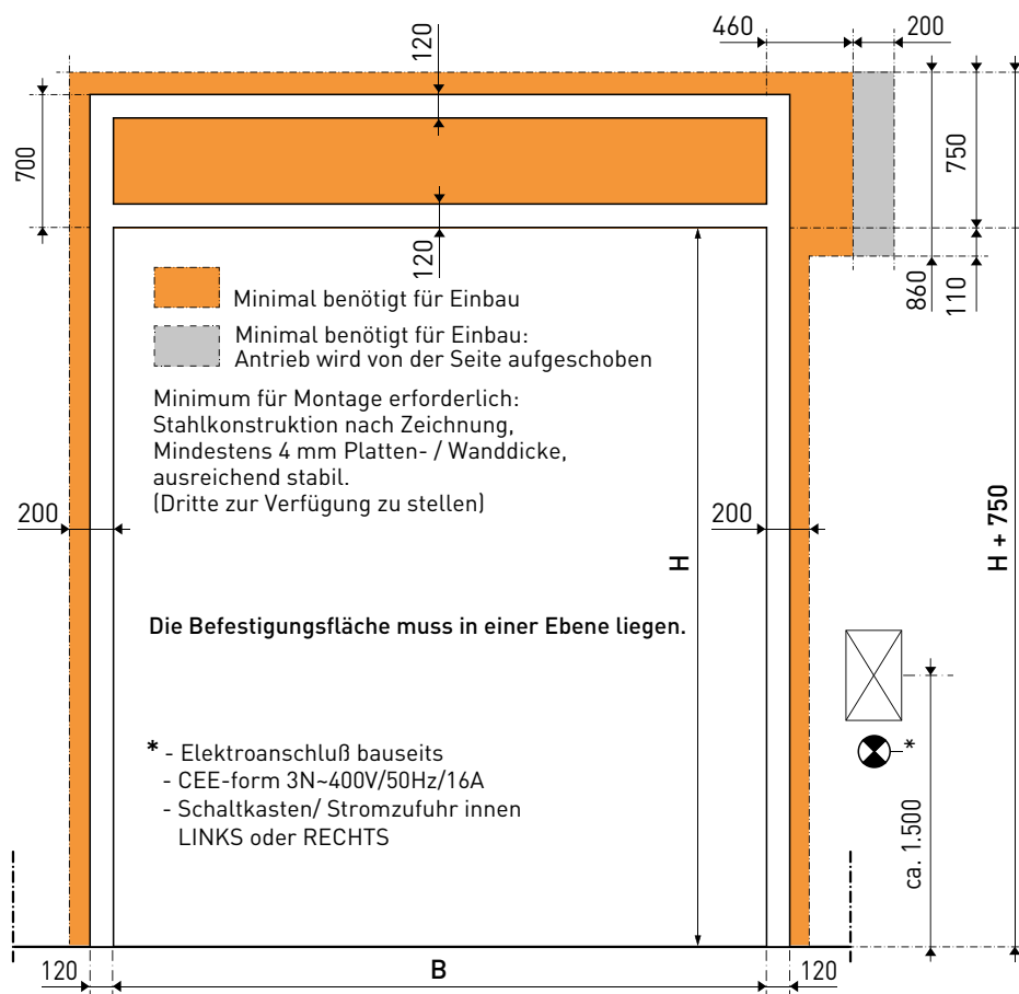
■ [ Vorderansicht ]
