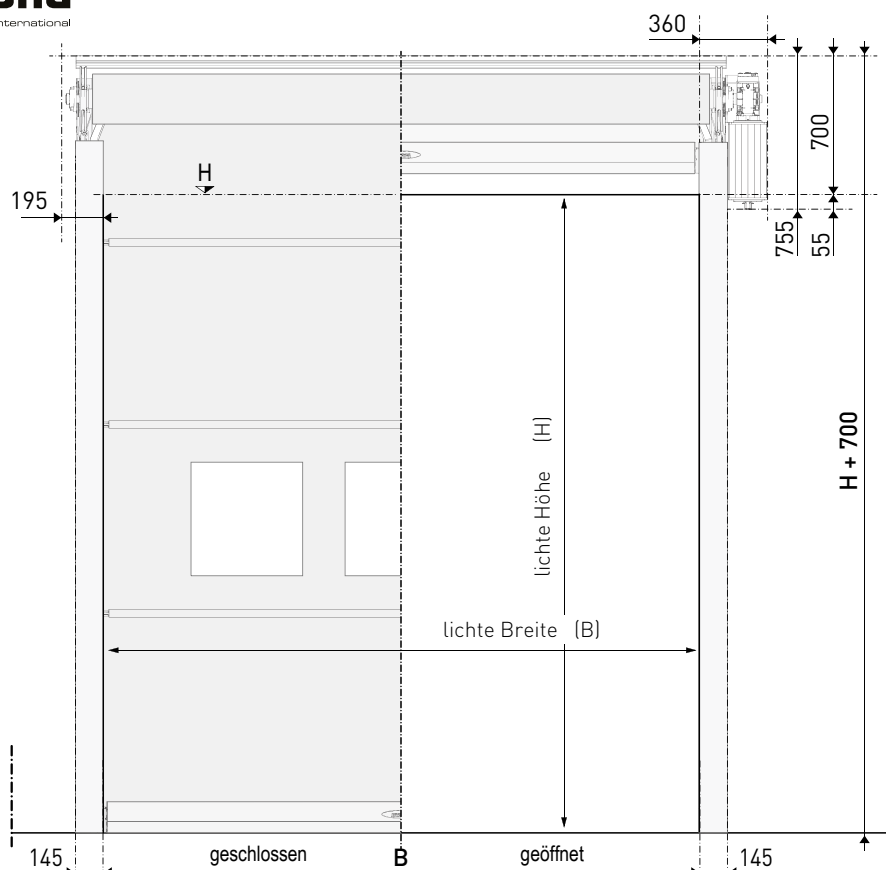
=[ Vorderansicht ]
